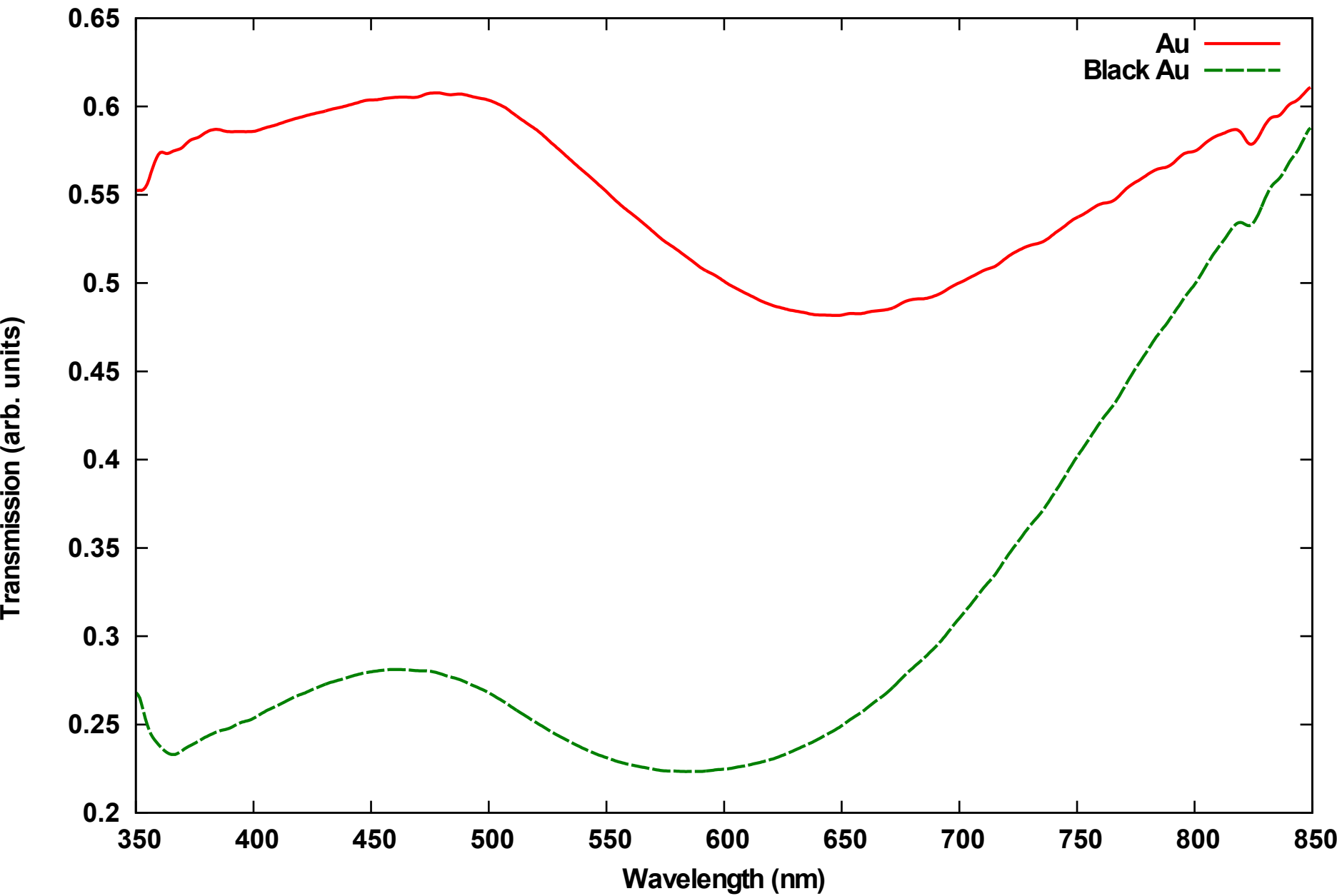
Transmission of Au and Black Au
